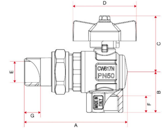
Рис.1 Чертеж с указанием размеров Fig.1 Drawing with dimensions
